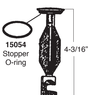
47041 Delrin stopper
